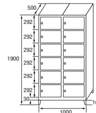
SB-50/2 COD. 45062
