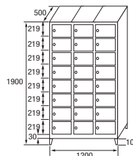
SZ-40/3 COD. 44083
