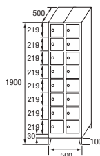
SZ-25/2 COD. 42582
