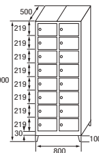
SZ-40/2 COD. 44082
