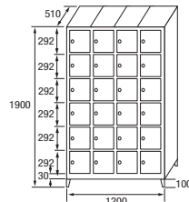
SB-30/4 COD. 43064
