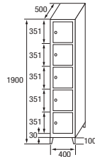
SP-40/1 COD. 44051
