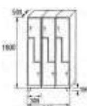
SL2-30/3 COD. 43043
