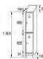
ST-40/1 Inox COD. 84911
