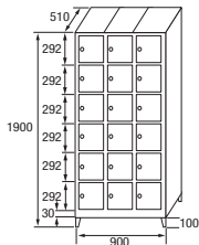
SB-30/3 COD. 43063
