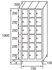
SB-25/3 COD. 42563
