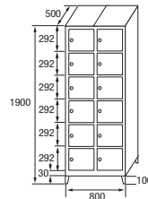
SB-40/2 COD. 44062
