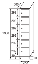
SB-40/1 COD. 44061
