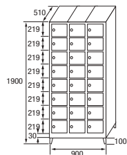
SZ-30/3 COD. 43083
