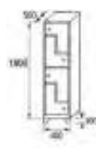
SL4-40/1 COD. 43054
