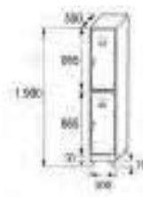
ST-30/1 COD. 43011
