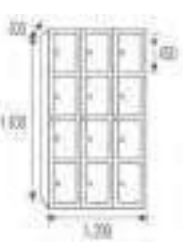
STV4-40/3 COD. 44843
