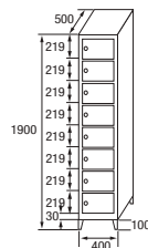
SZ-40/1 COD. 44081
