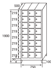
SZ-25/3 COD. 42583
